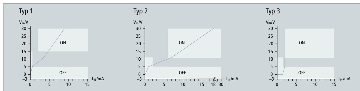
Abb. 3 Kennlinien der drei Eingangstypen (24 V DC) von Beckhoff
