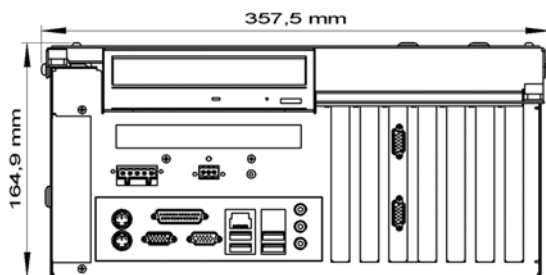
Frontansicht
