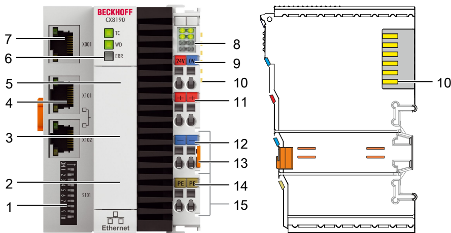
Abb. 1: Beispielaufbau eines Embedded-PCs CX8190.
