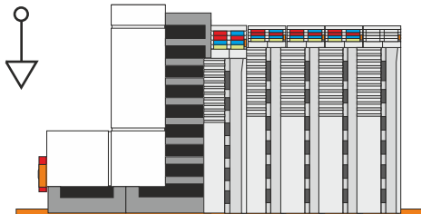
Abb. 7: Embedded-PC CX8190, liegende Einbaulage.
