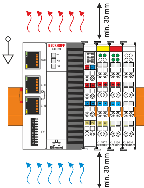
Abb. 5: Embedded-PC CX8190, waagerechte Einbaulage.
