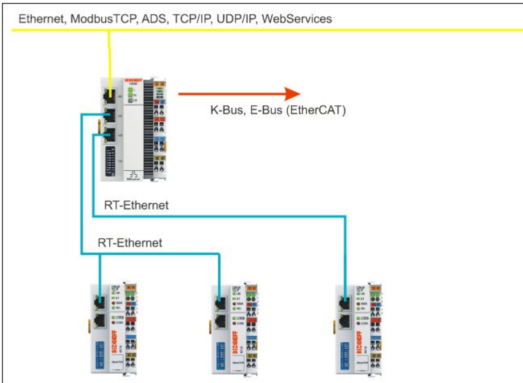
Abb. 14: Topologiebeispiel, CX8190 verbunden mit dezentralen Buskopplern über Realtime-Ethernet.
