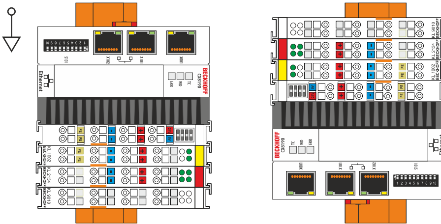
Abb. 6: Embedded-PC CX8190, senkrechte Einbaulage.
