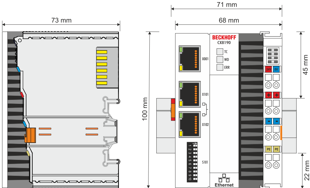
Abb. 4: Abmessungen des Embedded-PCs CX81xx.
